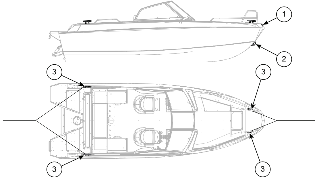
Abbildung 5.5 Buster XL/XXL Befestigungs- und Schlepppunkte
