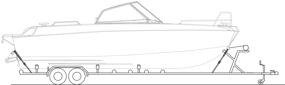
Abbildung 12.1 Buster XL/XXL Anhängertransport
