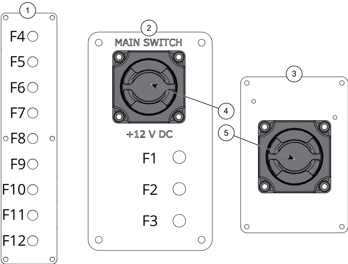
Abbildung 8.1 Buster XL/XXL-Hauptschalter und -Sicherungspanel
