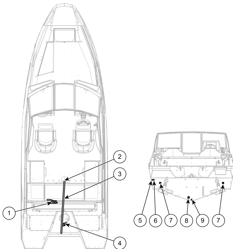
Abbildung 9.1 Buster XL/XXL Entwässerungsgerät
