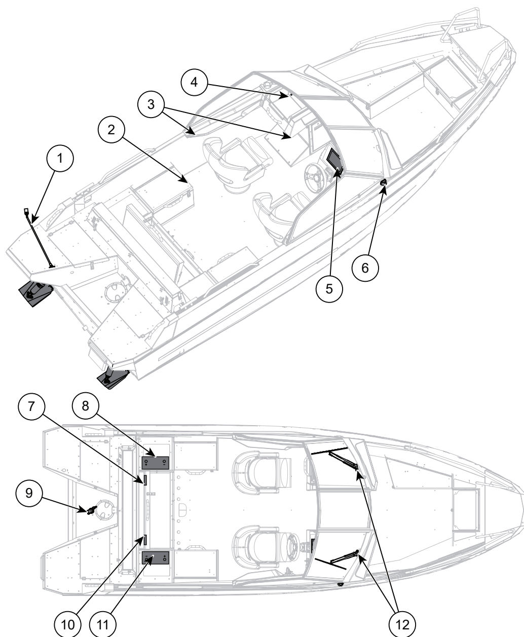
Abbildung 8.3 Buster XL/XXL Elektrische Ausrüstung
