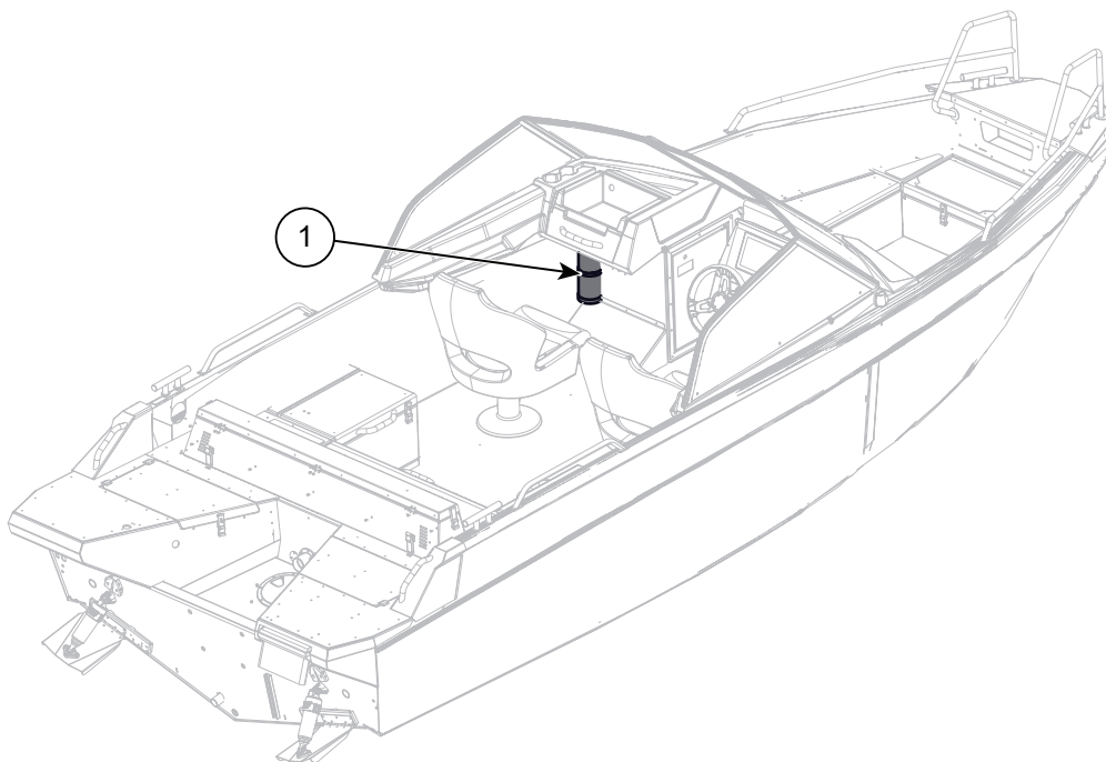
Abbildung 2.2 Buster XL/XXL Standort des Feuerlöschers
