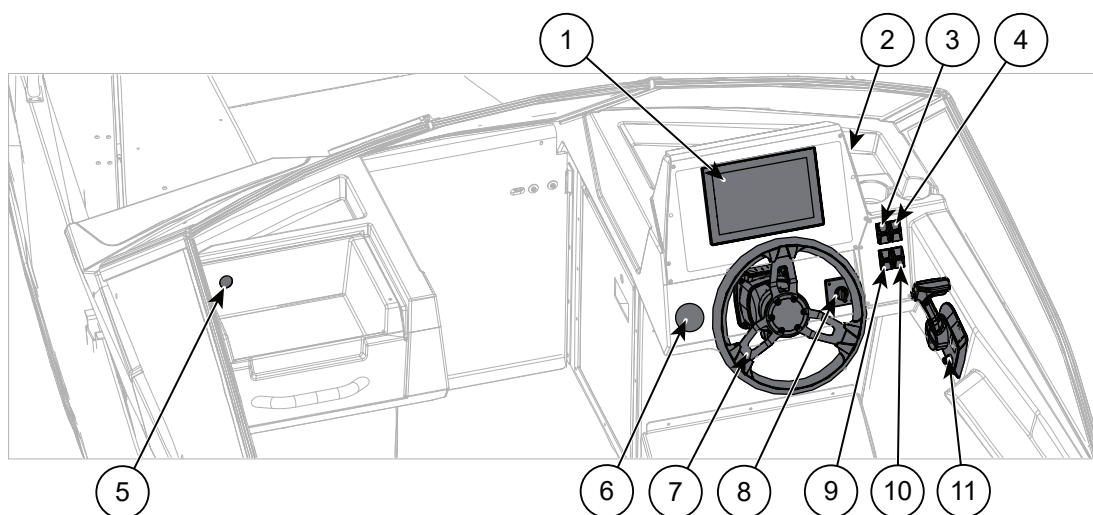
Abbildung 5.1 Buster XL/XXL Bedienelemente am Steuerstand
